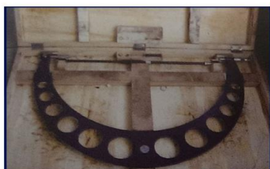
تجهیزات آزمون F7 (که برای میلگرد استفاده میشود)
